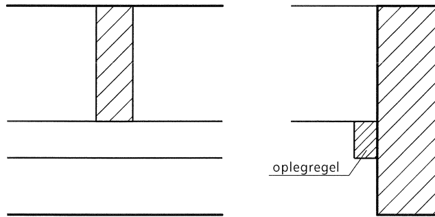
Detail 0504 met oplegregel
