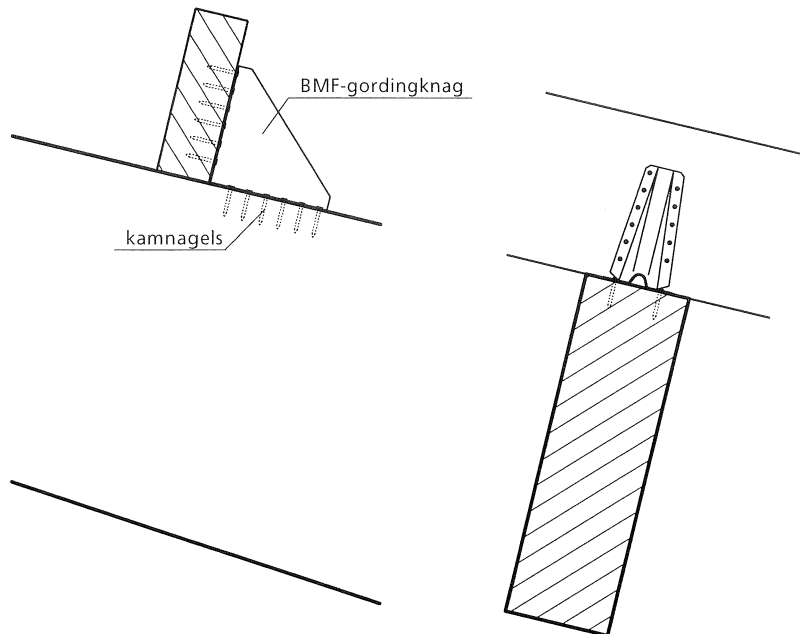
Detail 0505 met gordingknag
