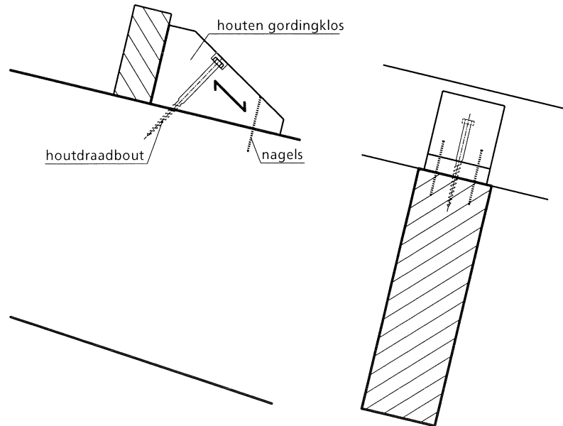
Detail 0506 met houten gordingklos
